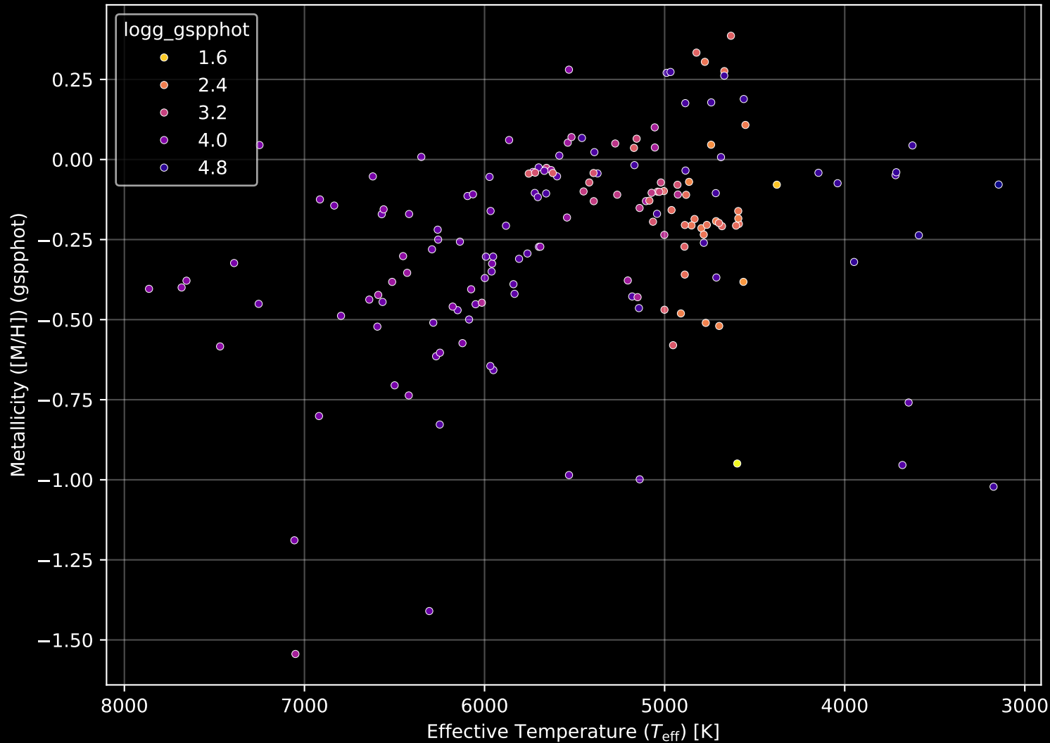
APOGEE DR17 Field: [CVZTILE_107+30_btx] Stellar Population Parameters (n= 166)
